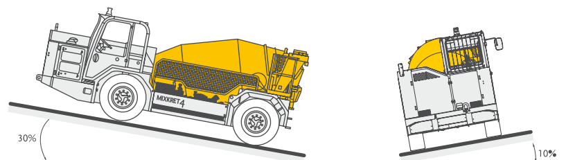
INCLINAÇÃO MÁXIMA LONGITUDINAL EM TRANSLAÇÃO
