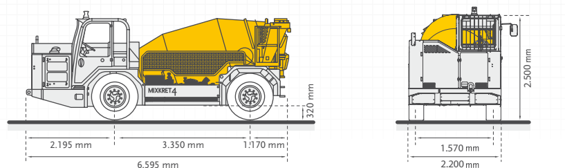
DIMENSÕES DE TRANSPORTE
